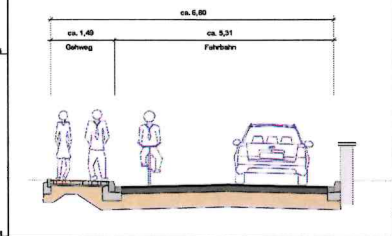
Systemquerschnitt Bestandsausbau
