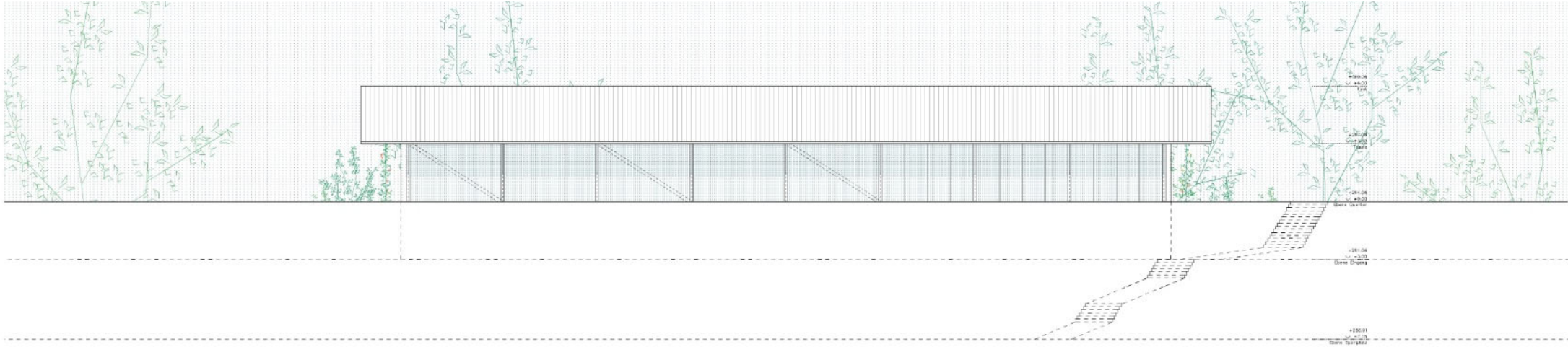
Ansicht Süd M1:100
