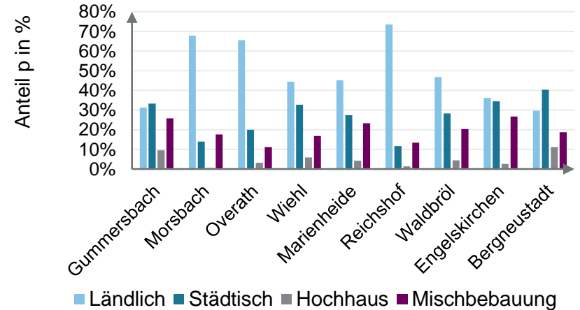
Anteil am Wärmebedarf 2020
