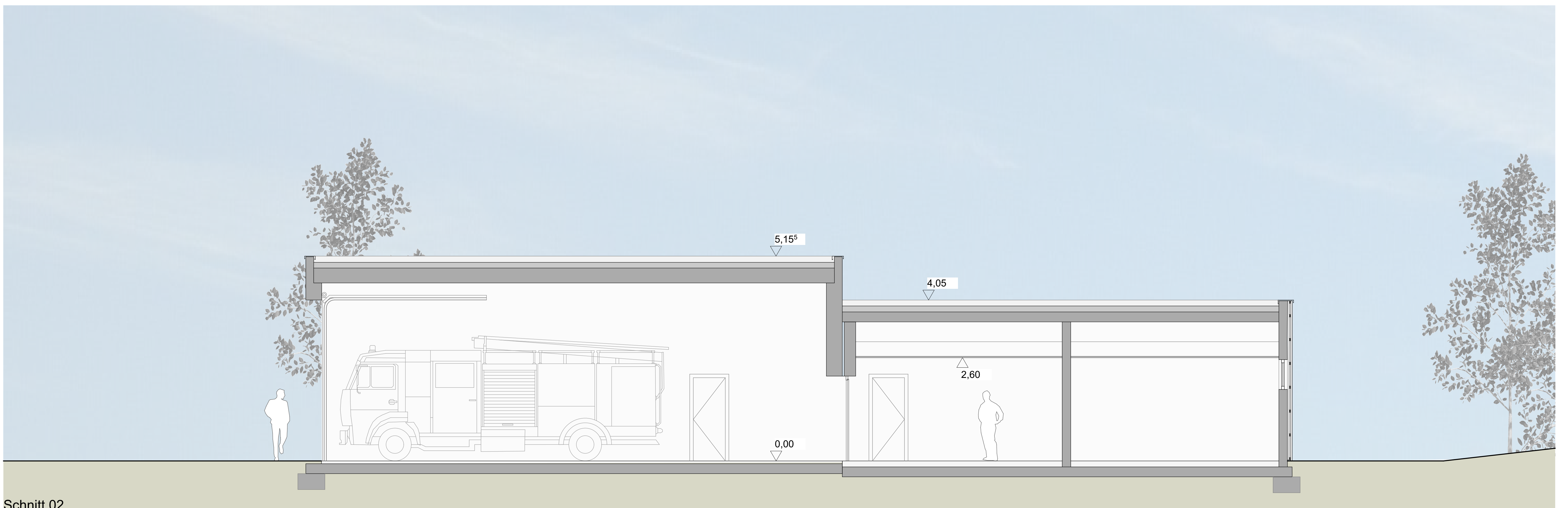
Schnitt 02
