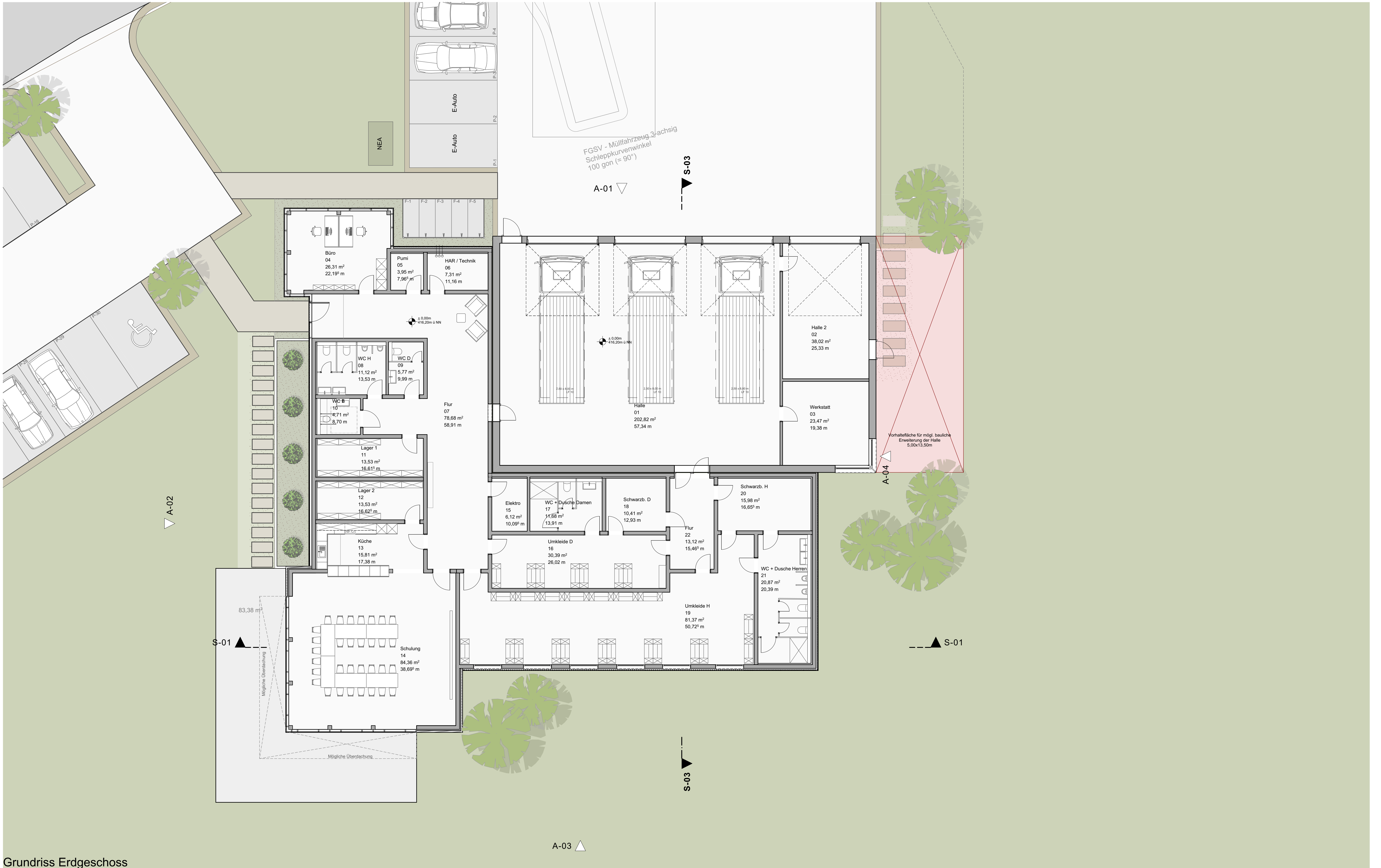
Grundriss Erdgeschoss
