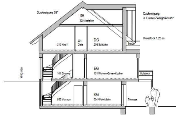
Haus Braun-Schönen Vorentwurf Schnitt A-A M 1:100 08.10.2021
