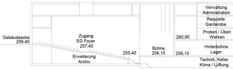
Schnitt A-A
